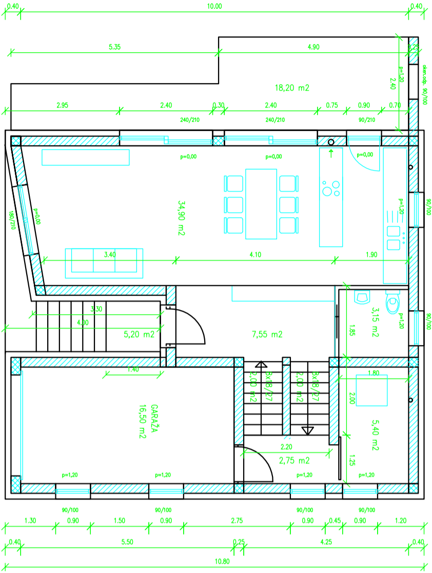
TLORIS PRITLŪČJA
