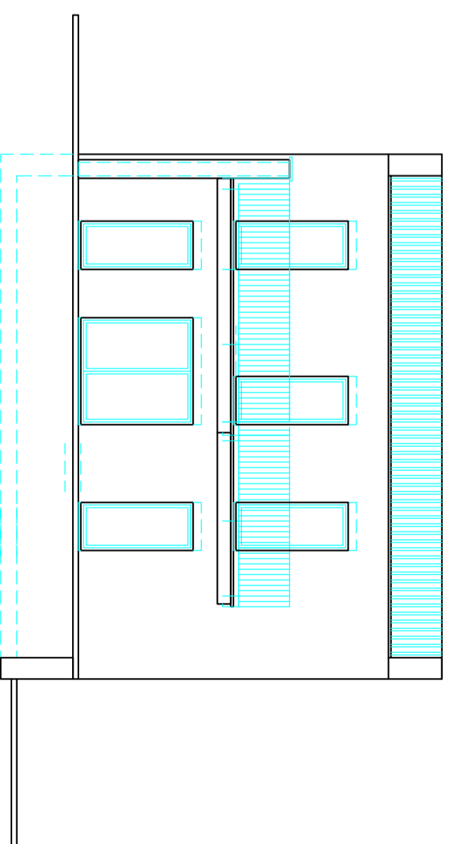
ZAHODNA FASADA
